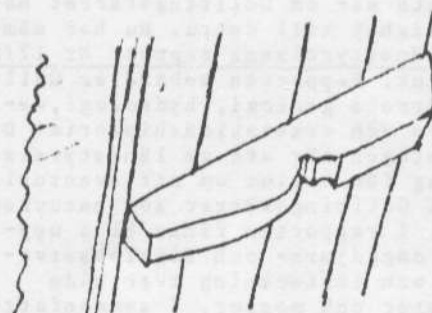
Utskjutande takspärre
